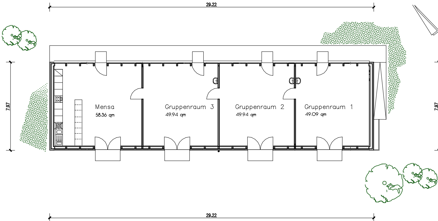
GRUNDRISS
