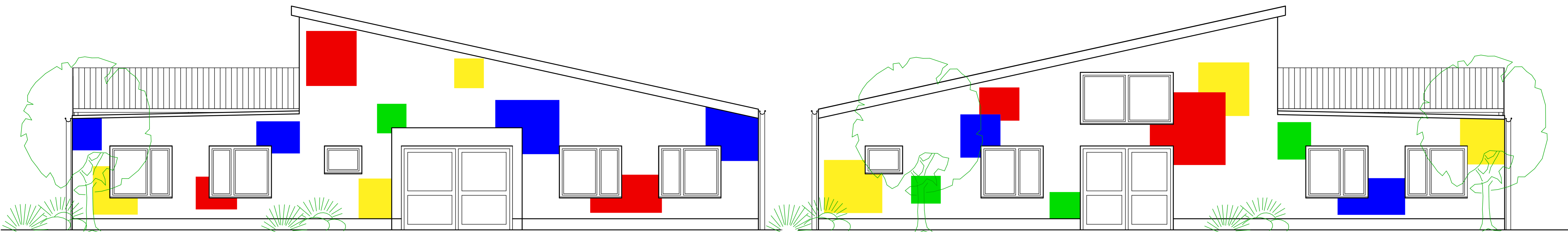
WESTANSICHT
