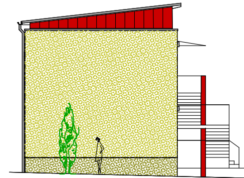
OSTANSICHT
